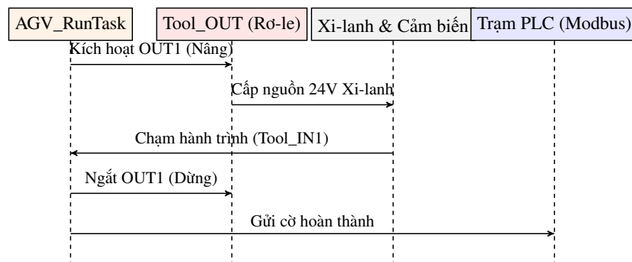
Hình 4.10 Sơ đồ tuần tự hoạt động của cơ cấu móc kéo xe hàng.
