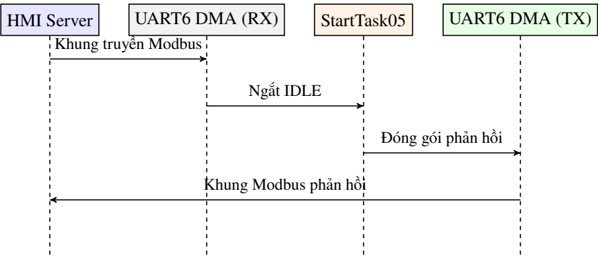
Hình 4.12 Sơ đồ tuần tự giao thức truyền thông Modbus RTU.
