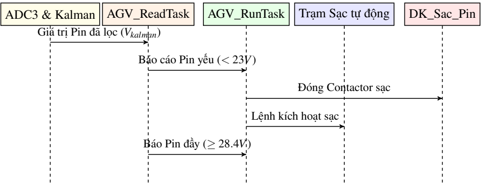
Hình 4.11 Sơ đồ tuần tự quá trình giám sát Pin và sạc tự động.
