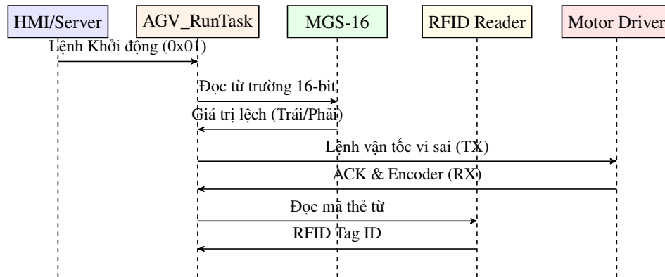
Hình 4.8 Sơ đồ tuần tự quá trình dẫn đường và nhận dạng trạm RFID.
