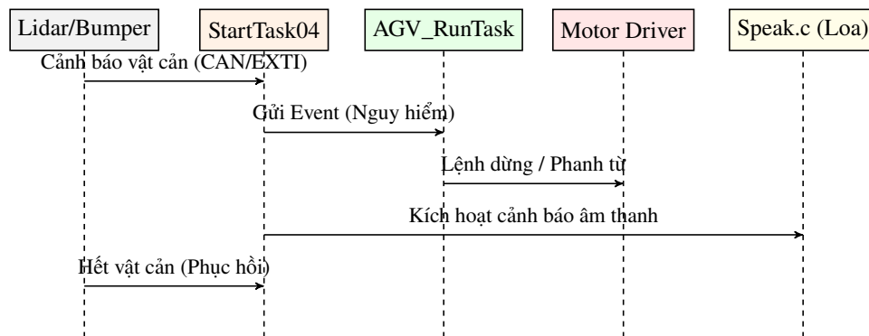
Hình 4.9 Sơ đồ tuần tự luồng giám sát an toàn và xử lý sự cố.
